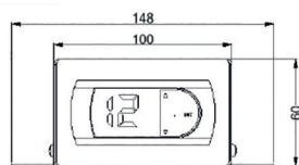
Skříňka termostatu boční pohled:
