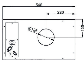
Skříňka termostatu čelní pohled:
