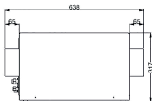
Vnitřní jednotka boční pohled:
